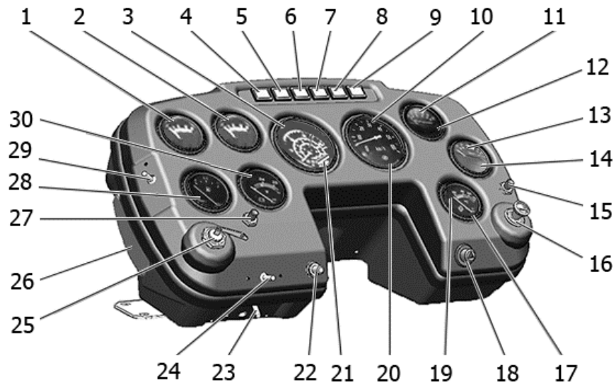
Рисунок 9 – Панель приборов
