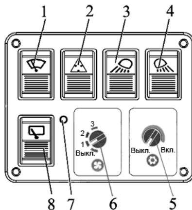
Рисунок 8 – Панель переключателей
